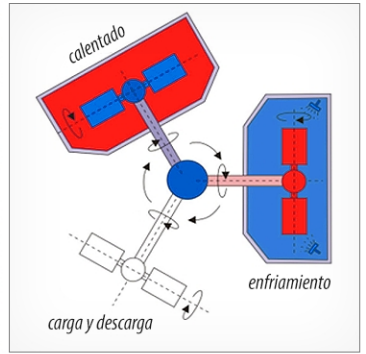
Moldeo rotacional
