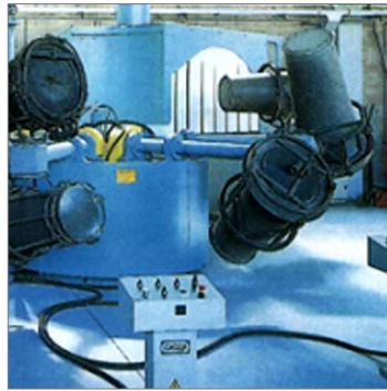
Moldeo rotacional
